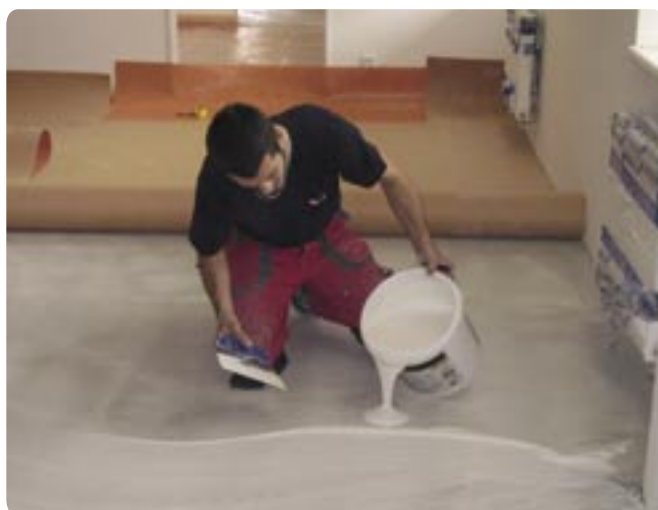
Lepení přírodního linolea pomocí lepidla na linoleum LKL 334.
