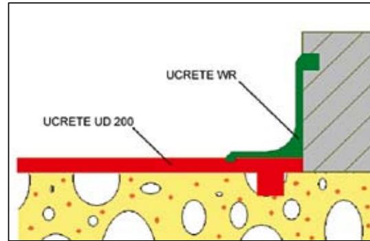
Obr. 1 Fabion - alternativní řešení
