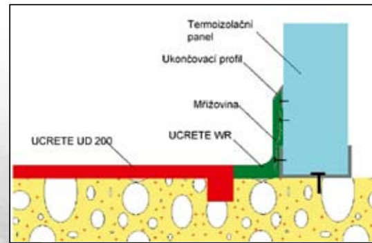
Obr. 3 Fabion u termoizolačního panelu
