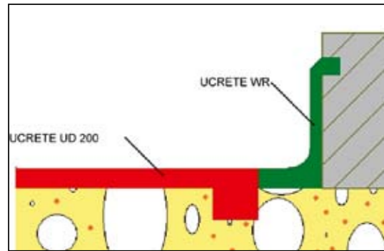
Obr. 2 Fabion - doporučené řešení
